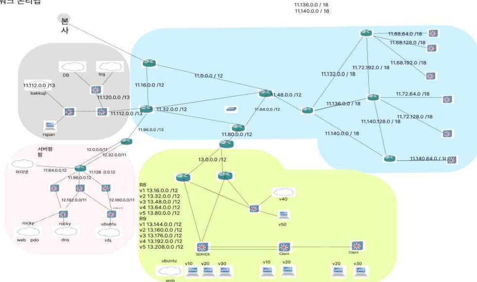
네트워크 논리맵
